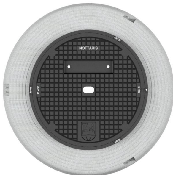
Fig. 3901-60-10 AT stufenlos höhenverstellbar mit Pickelloch
